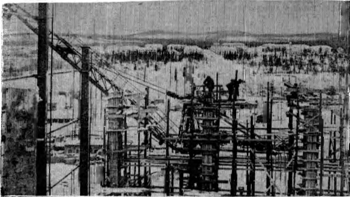
ПОСЕЛОК КОВДОР. На снимке: бетонирование колонн по оси «Д» на корпусе сушики. Фото М. Меламуда, инженера-геодезиста треста «Ковдорстрой»
