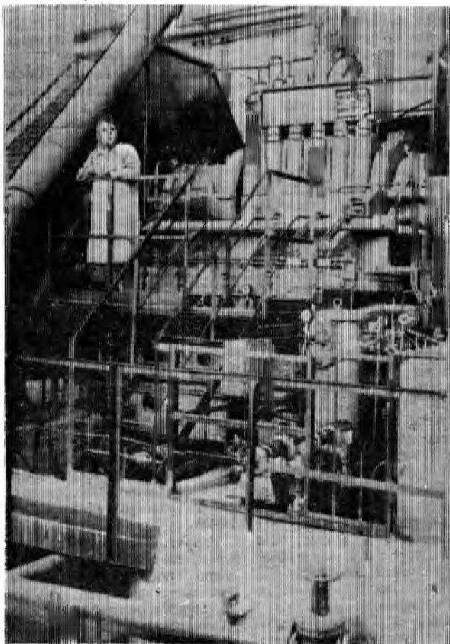
ПОСЕЛОК КОВДОР. Щековая дробилка отделения крупного дробления обогатительной фабрики.
