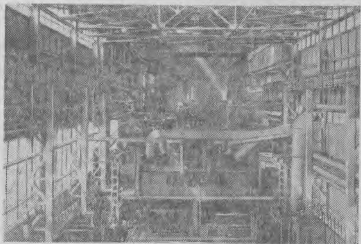
На Руставском металлургическом заводе завершено сооружение нового агрегата мартеновского цеха — установки непрерывной разливки стали (на снимке). По высоте она равна пятиэтажному дому, длина ее 150 метров.
