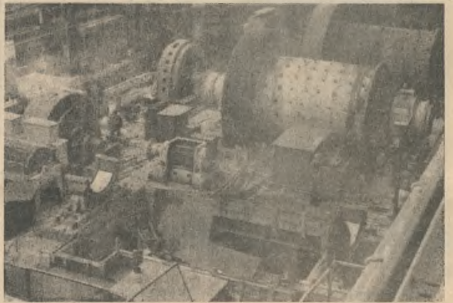
Так быстро меняется ситуация на площадке, что трудно на газетном снимке показать, что происходит на шестой секции в данный момент. Фотографии чуть больше недели, а картина изменилась значительно. Уже поставлена на место и вторая мельница. Монтаж оборудования продолжается.
