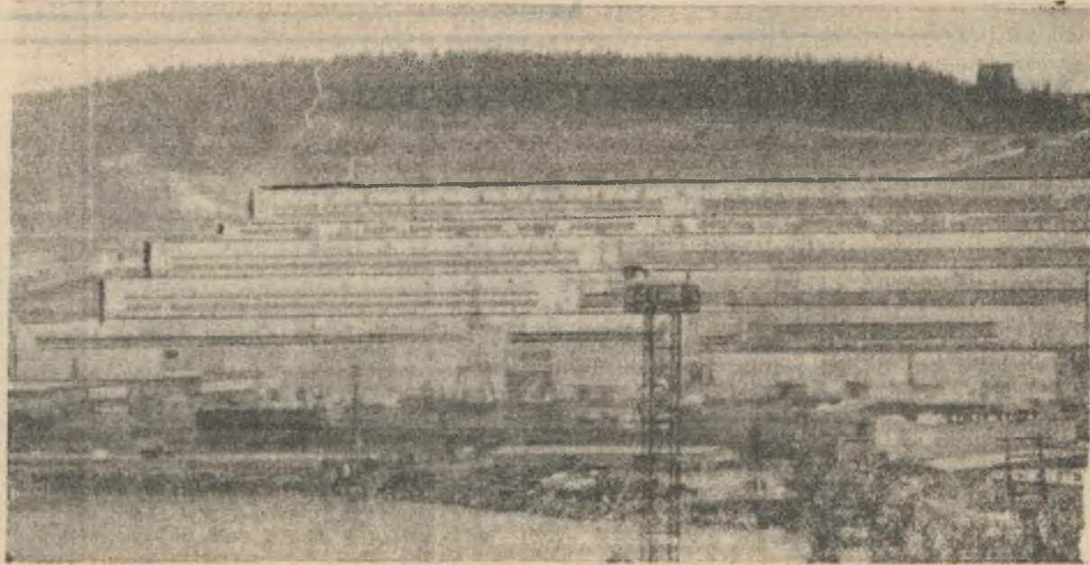
Апатито-бадделитовая обогатительная фабрика Ковдорского горно-обогатительного комбината — первенец на пути комплексного использования сырья Ковдорского
