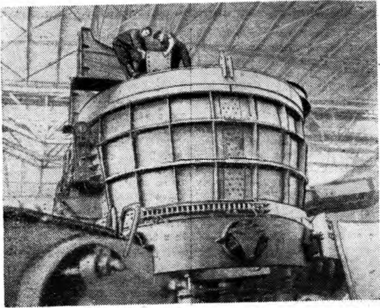
На Новосибирском заводе электротермического оборудования изготовлена новая 25-тонная электросталеплавильная печь. В отличие от существующих она имеет отворачивающийся свод. Это позволяет механизировать ее загрузку. Печь предназначена для Уралмашзавода.
